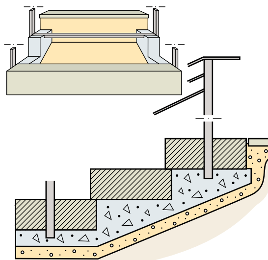
Fig 7.30 Räcke monterat i ett infästningsstål under blockstegen, som är monterade på långsgående balkar.
