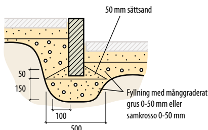
Fig 6.15 Typkonstruktion KG
