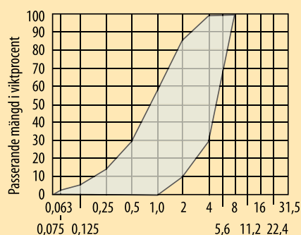
Fig 3.5 Siktkurva, sand för sättning och fogning av plattor och gatsten.
