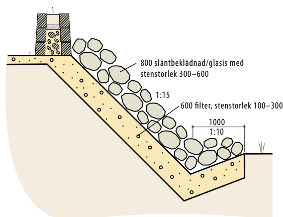
Fig 8.39 Släntbeklädnad med av fältstenar.
