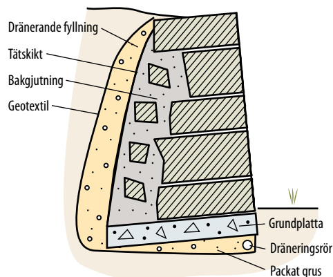
Fig 8.33 Bruksmur av block med bakgjutning. Typkonstruktion M4
