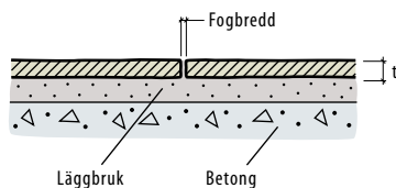
Fig 4.21 Läggning av hällar i bruk på underlag av betong.
