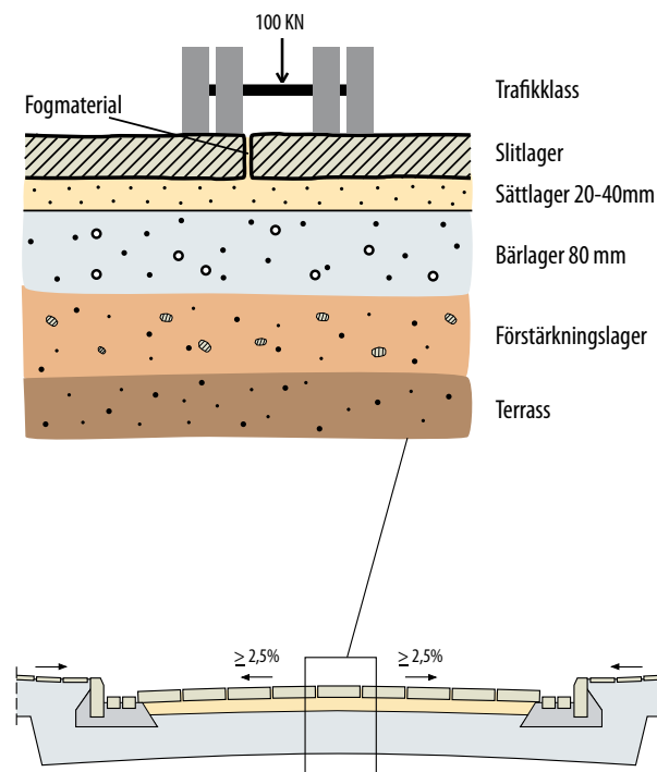
Fig 4.32 Uppbyggnad av vägbana belagd med hållar. Kantsten som motstöd.
