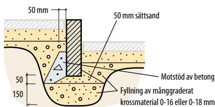
Fig 6.17 Typkonstruktion KG
